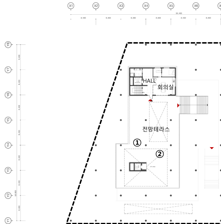
3층평면도
